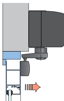
Trekend armsysteem Type PULL
