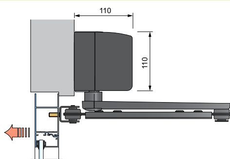
Duwend armsysteem Type PUSH
